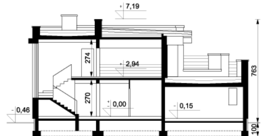
Przekrój
