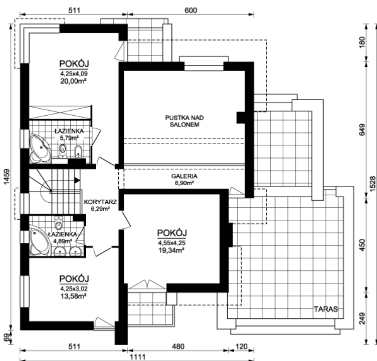
Rzut piętra
