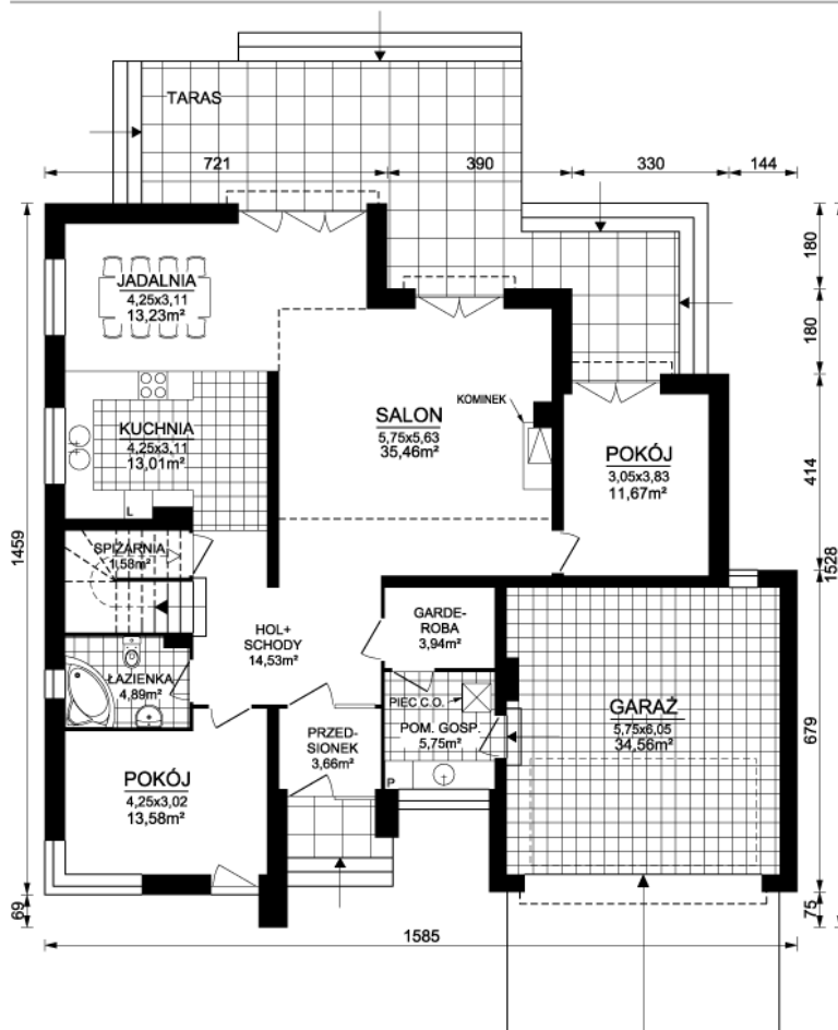
Rzut parteru
