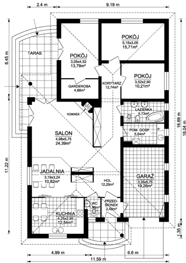
Rzut parteru
