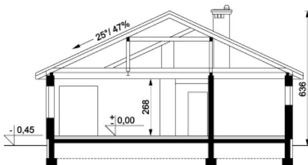
Przekrój
