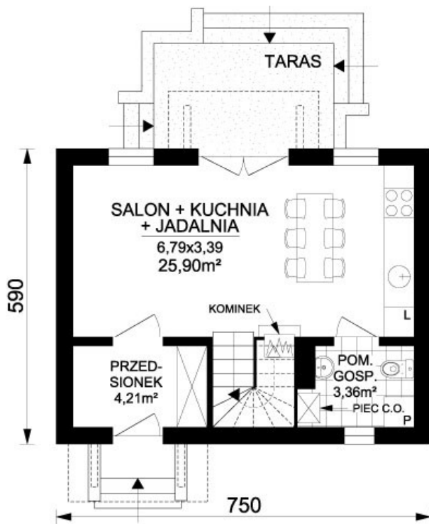
Rzut parteru
