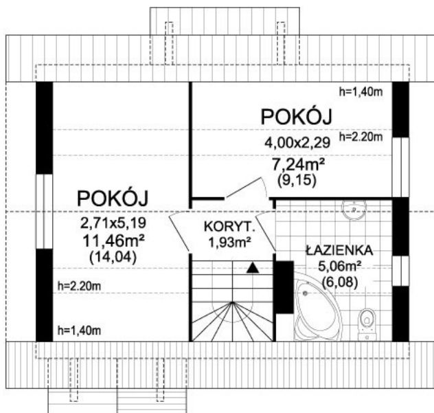
Rzut poddasza
