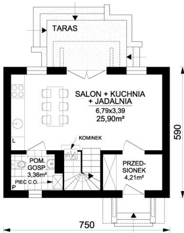
Rzut parteru
