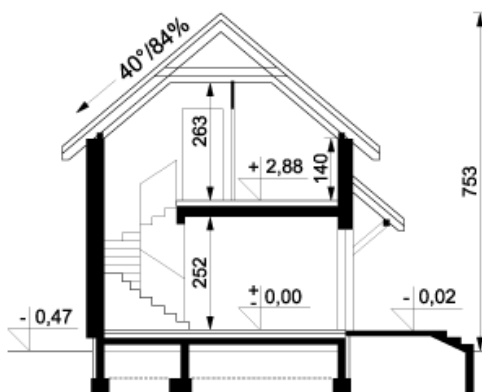
Przekrój
