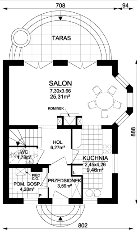
Rzut parteru
