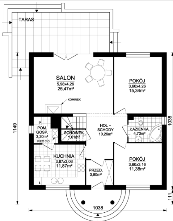
Rzut parteru
