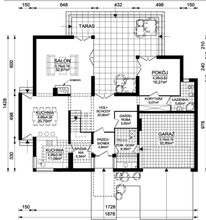
Rzut parteru
