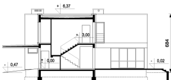
Przekrój
